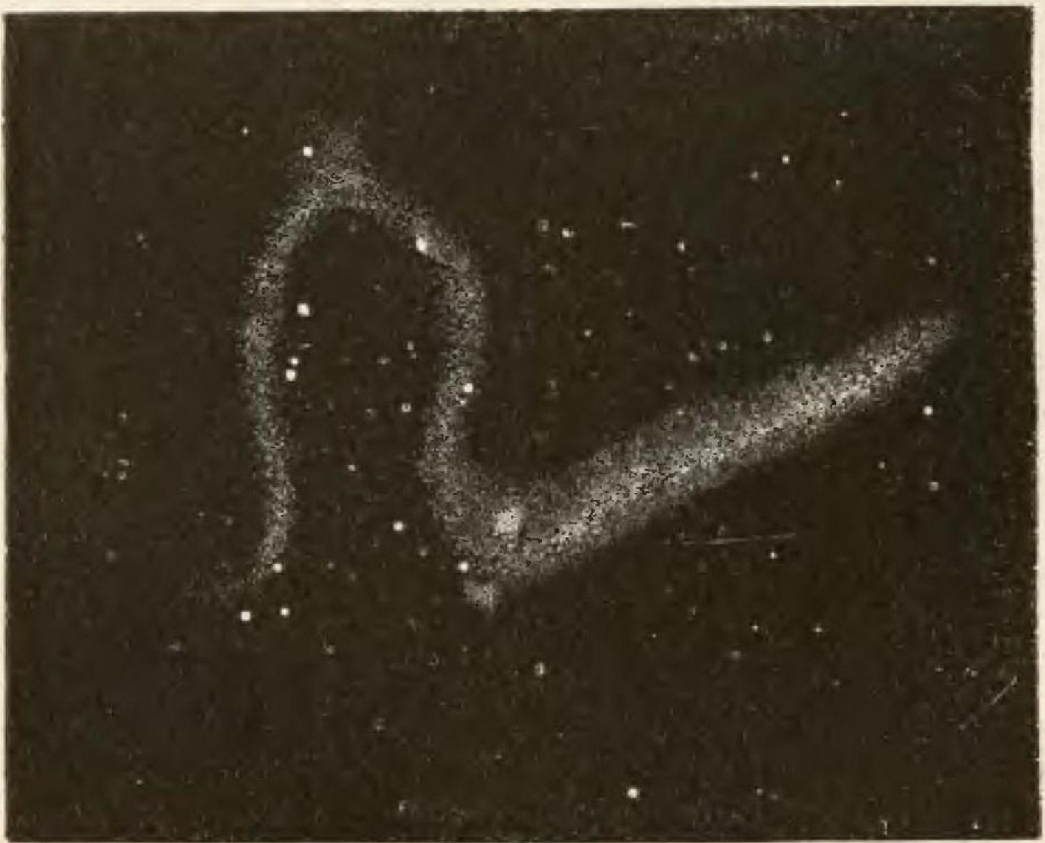
FIG. 1.—J. HERSCHEL, 1833.
